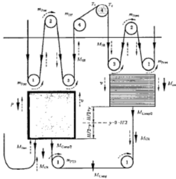
1,2,3,4—滑轮的速度系数(例如,2表示2·v 轿厢 )
