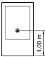
d) 具有较大玻璃面板 或全玻璃的层门
