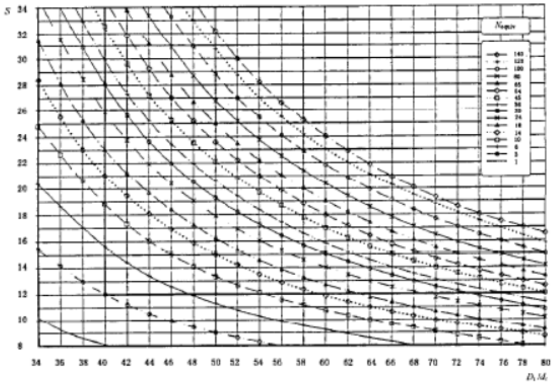
图 N1 最小安全系数的计算
