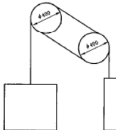
图 N2 滑轮等效数量的计算示例
