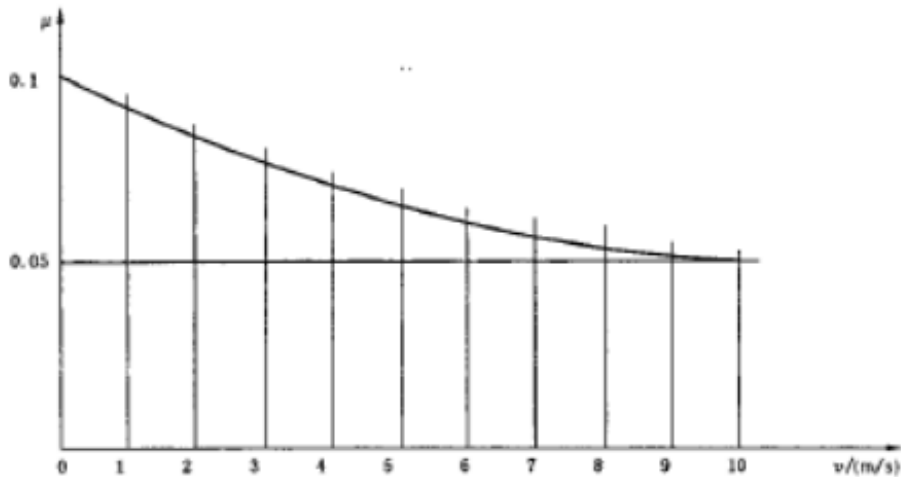
图 M3 最小的摩擦系数
