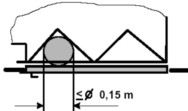
图5 铰链层门和折叠轿门的间隙
