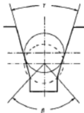
图 M2 V形槽
