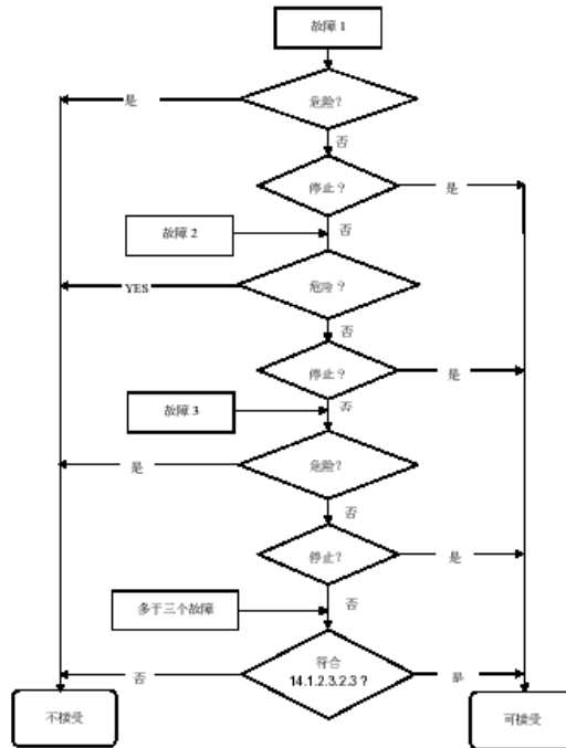
图6安全电路评价流程图
